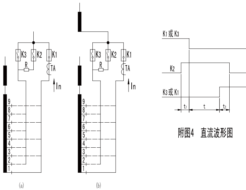
附图3 分接开关工作原理图
