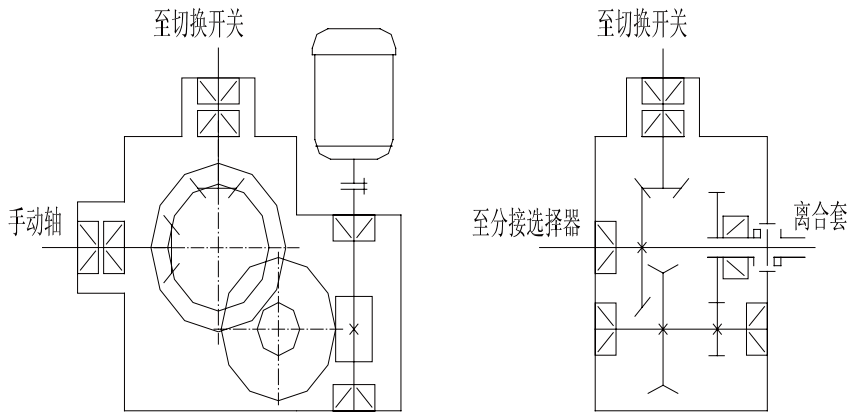
附图2 减速箱传动示意图
